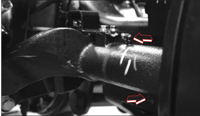
5) 리어 챔버브라켓 및 슬랙어저스터(드럼 브레이크 적용차량)
