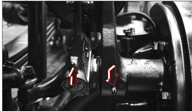
4) 프론트 챔버브라켓 및 슬라이져스트(드럼 브레이크 적용차량)
