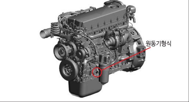
CURSOR 9(FPT) 엔진
