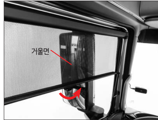
사이드 선바이저를 올릴때는 가이드바를 안쪽으로 잡아당겨 올려 주십시오.
