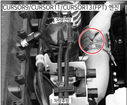
1) CURSOR 9/CURSOR 11/CURSOR 13(FPT) 엔진 : 캡을 올리면 오른쪽(조수석쪽) ECU 상단부에 게이지가 있습니다.
