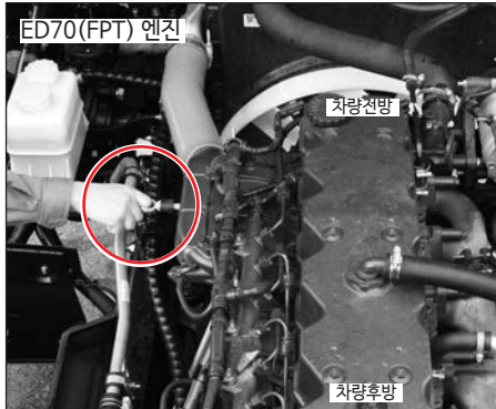
2) ED70(FPT) 엔진 : 캡을 올리면 엔진 왼쪽(운전석 쪽) ECU 상단부에 게이지가 있습니다.
