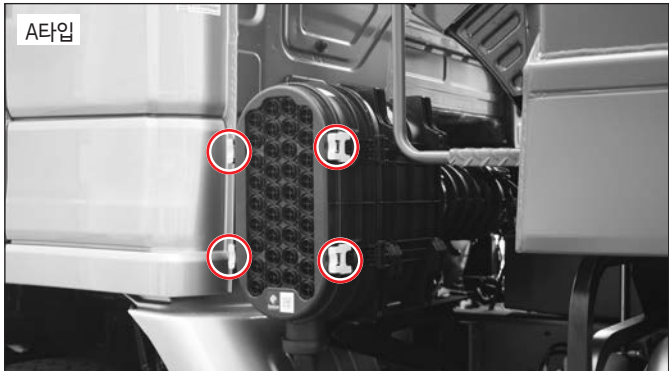
1) 4개 또는 6개의 클램프를 풀어 에어클리너 뚜껑을 열고 엘리먼트를 탈거하십시오.
