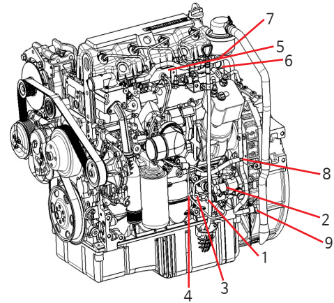
F4.5(CUMMINS)엔진
