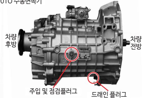
ZF6S1000TO 수동변속기
