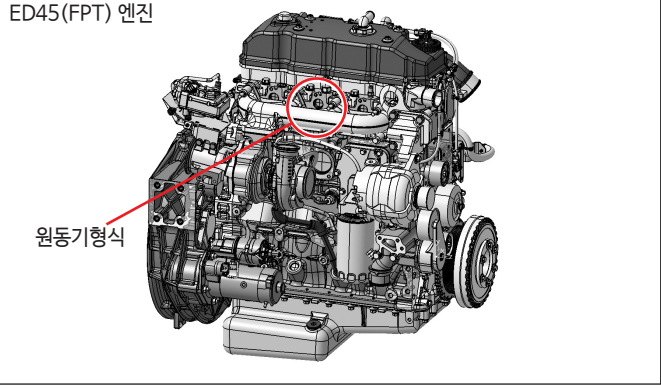
ED45(FPT) 엔진
