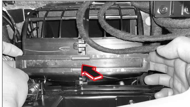
4. 새로운 에어 필터를 제공되어 있는 슬롯에 끼운 후 밀어서 단단히 잠급니다. 5. 퓨즈박스 커버를 닫으십시오.
