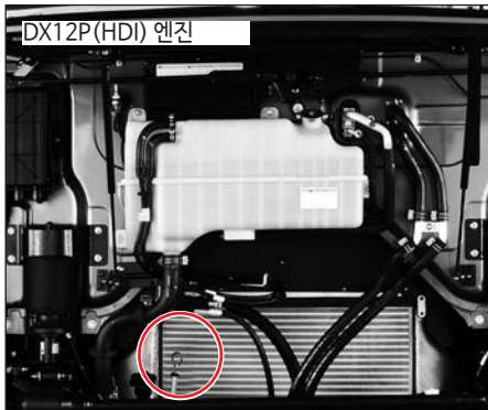
3)DX12P(HDI) 엔진 :앞 점검 판넬을 당겨서 열면 라디에이터 앞쪽에 게이지가 있습니다.
