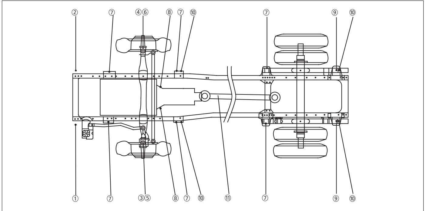
(1) 4×2차량 새시그리스 주입도
