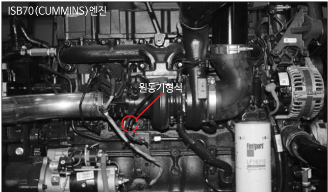
ISB70(CUMMINS) 엔진은 실린더블럭 우측 하단 중간쪽에 새겨져 있습니다.
