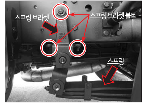
뒷쪽 스프링 브라켓 볼트 (운전석 3개소, 조수석 3개소)
