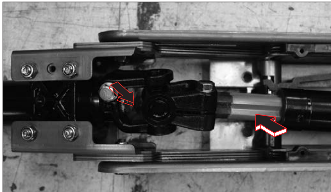
2) 스티어링 컬럼, 인터미디엇 샤프트의 스플라인 내부 및 U조인트 (위,아래)
