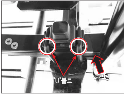
"U" 볼트
