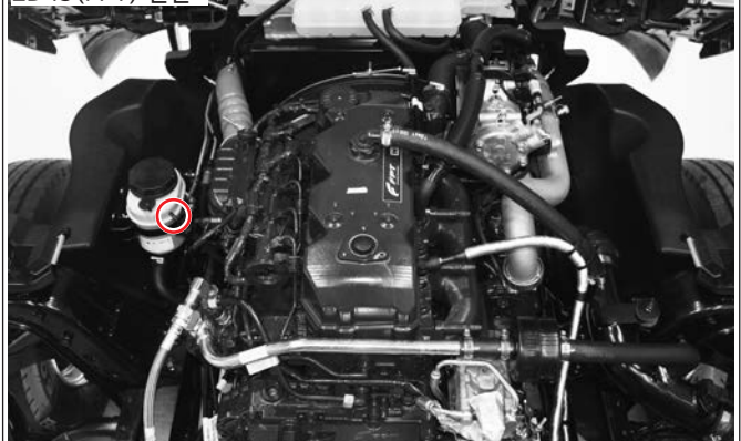
ED45(FPT) 엔진
