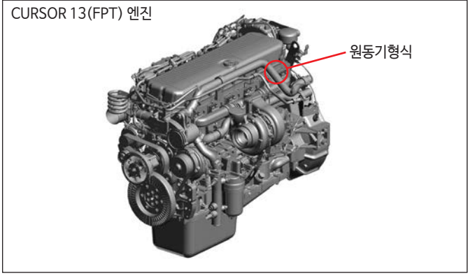
CURSOR 13(FPT) 엔진은 실린더블럭 좌측상단 뒤쪽에 새겨져 있습니다.
