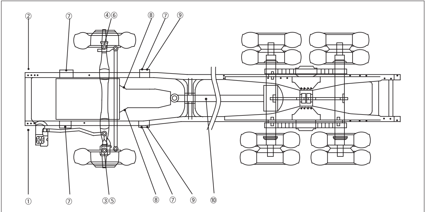
(2) 6X2, 6×4차량새시그리스 주입도
