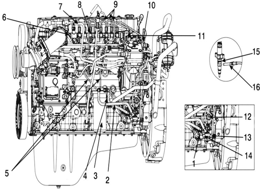
ISB70(CUMMINS)엔진
