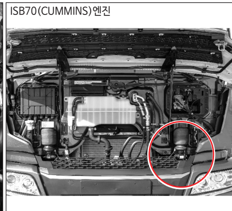
3) ISB70(CUMMINS) 엔진 : 앞 점검 판빌을 당겨서 열면 라디에이터 오른쪽에 게이지가 있습니다.
