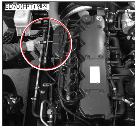
2) ED70(FPT) 엔진 : 캡을 올리면 엔진 왼쪽(운전석 쪽) ECU 상단부에 게이지가 있습니다.
