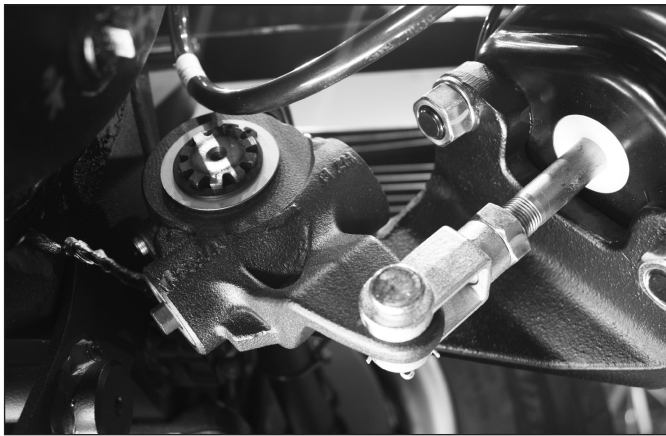
(2) 자동라이닝 조정장치 자동라이닝 간극조정 장치는 브레이크 라이닝 마모에 따른 간극조정을 자동으로 하는 장치입니다.
