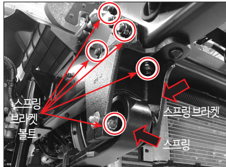
앞쪽 스프링 브라켓 볼트
