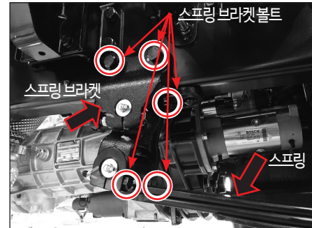
뒷쪽 스프링 브라켓 볼트
