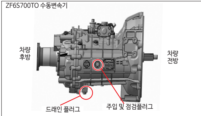
ZF6S700TO 수동변속기
