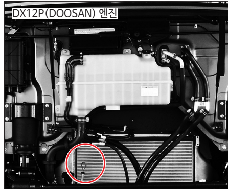
3) DX12P(DOOSAN) 엔진 : 앞 점검 판넬을 당겨서 열면 라디에이터 앞쪽에 게이지가 있습니다.
