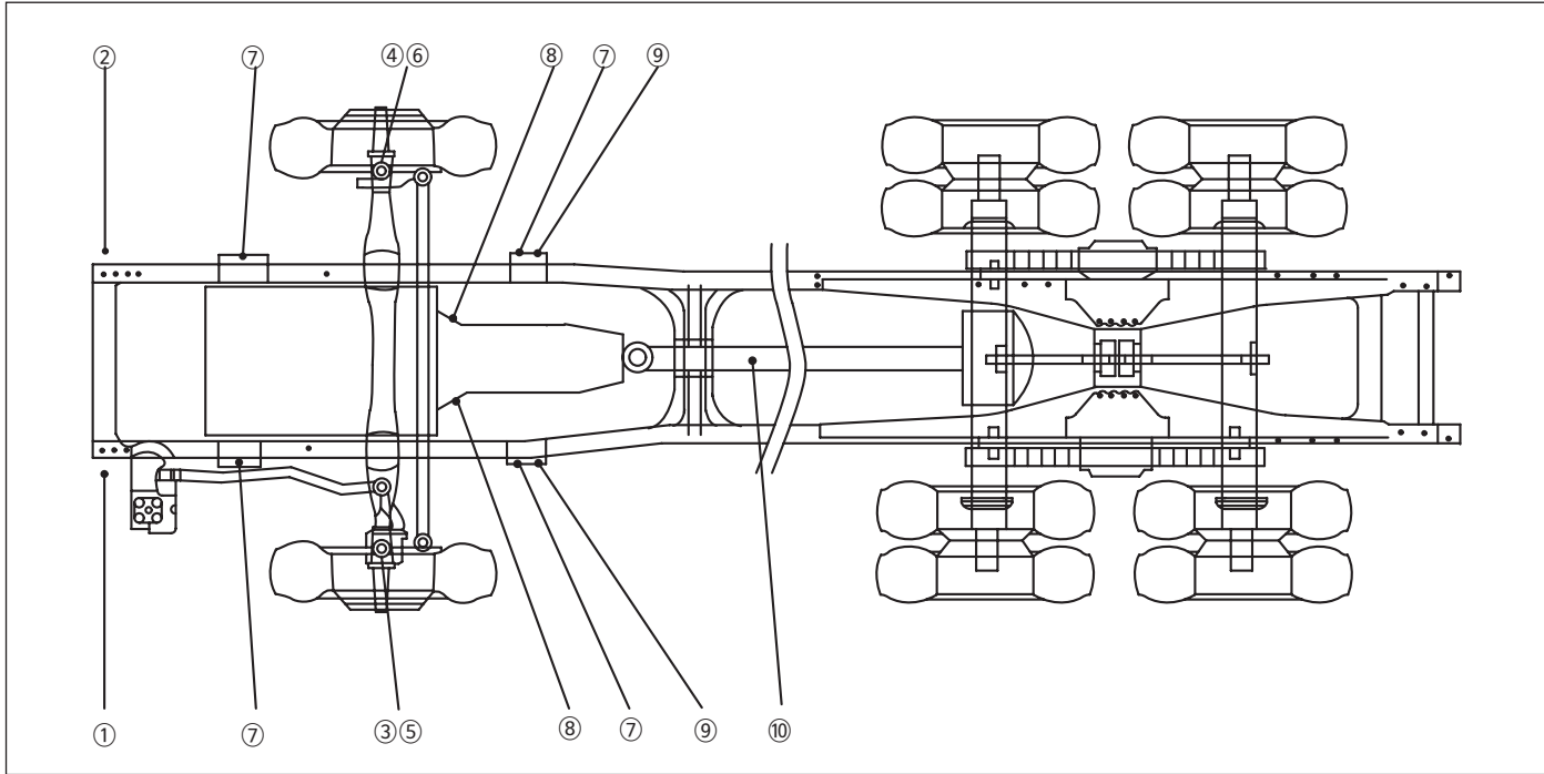
(2) 6X2, 6×4차량 샤프트그리스 주입도
