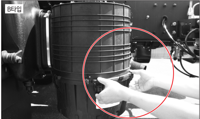
1) 6개의 클램프를 풀어 에어클리너 뚜껑을 열고 엘리먼트를 탈거하십시오.
