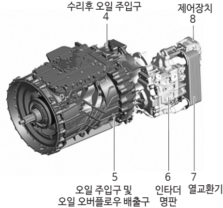
수리후 오일 주입구
