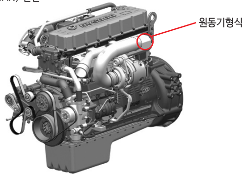
DX12P(DOOSAN) 엔진
