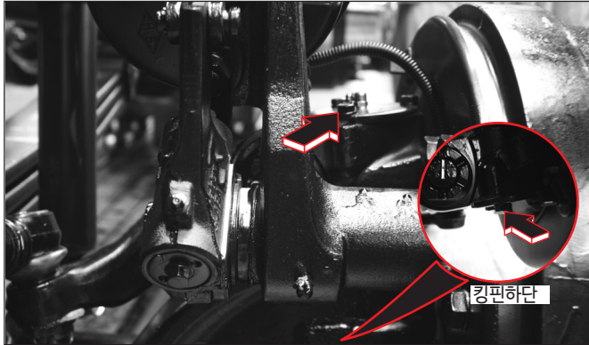
1) 킹핀
