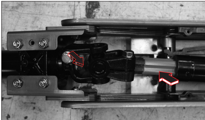
2) 스티어링 컬럼, 인터미디어트 샤프트의 스플라인 내부 및 U조인트 (위, 아래)
