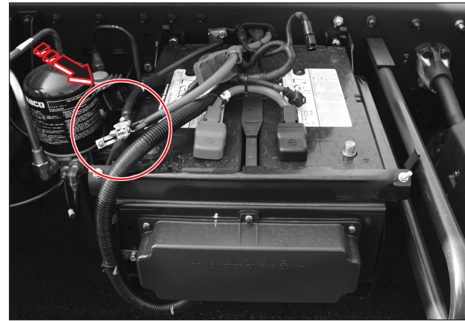
( 용접작업시 )
