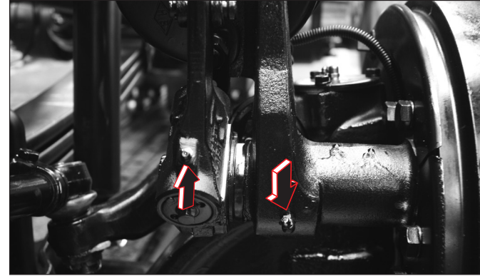
4) 프런트 챔버브라켓 및 슬랙어저스트
