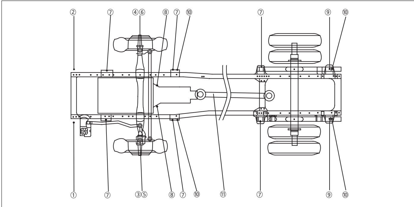
(1) 4×2차량새시그리스 주입도
