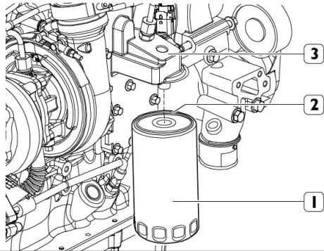
NEF(FPT) 엔진
