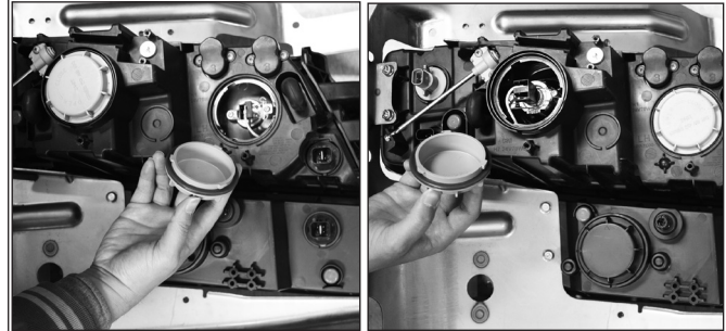
상향등 (H1)
