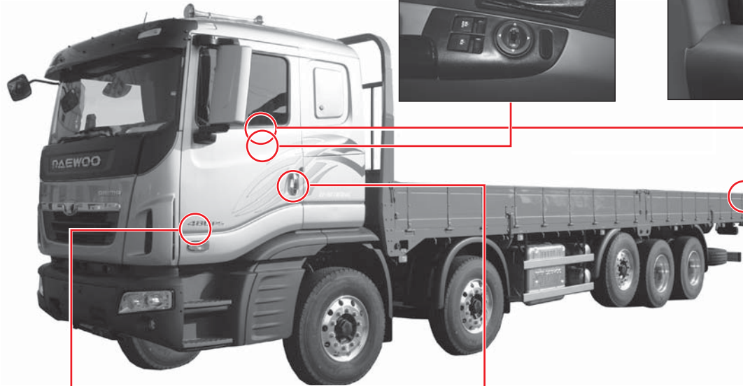
앞 점검판넬 열림 레버
