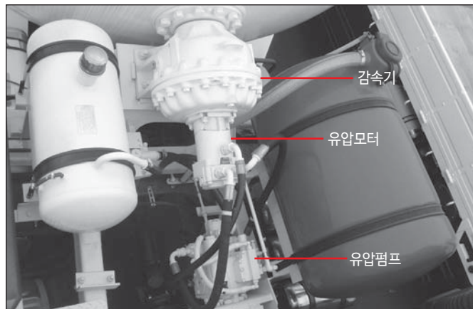
(4) 유압장치
