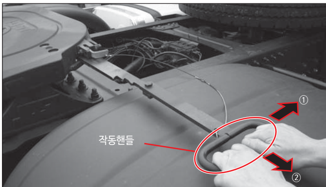
4) 커플러 작동핸들을 ①번 방향으로 이동하여 록킹 옛지로부터 작동핸들 걸림을 해제한 후 ②번 방향으로 완전히 당겨 주십시오.
