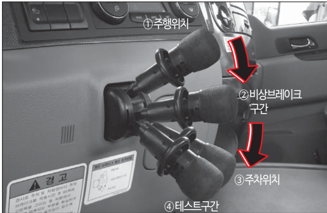
테스트 구간이 있는 주차브레이크 (트랙터, 풀카고 차량)
